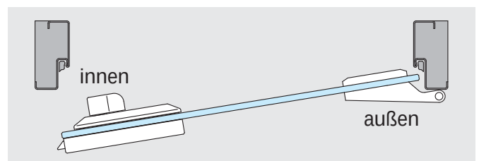
Bedienknebel auf Klemmplatseite ( DIN rechts auswärts )
