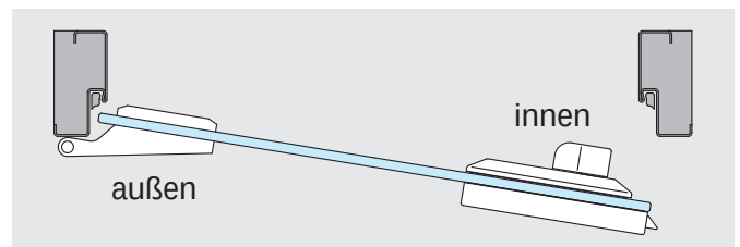
Bedienknebel auf Klemmplattemseite ( DIN links auswärts )
