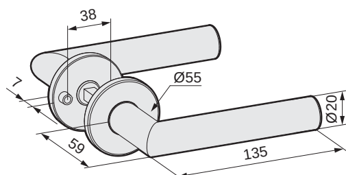
mit Drückerrosetten
