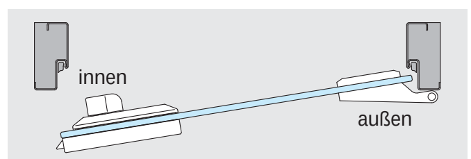
Bedienknebel auf Klemmplattemseite ( DIN rechts auswärts )
